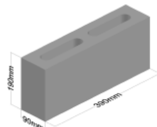
Hollow 100 390*190*90mm
