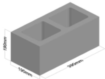
Hollow 200 390*190*190mm
